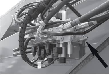
Fig. 8 Overdrukklep hoogwerkerdeel
