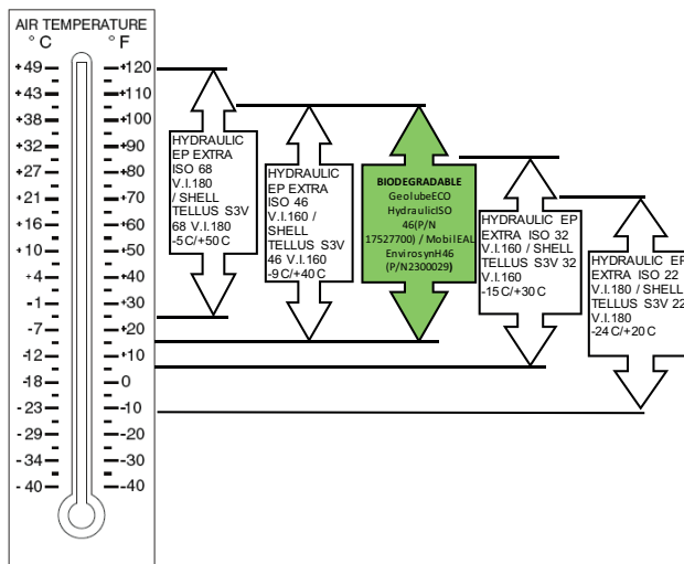
Fig. 119 Gebruikstemperaturen olie
