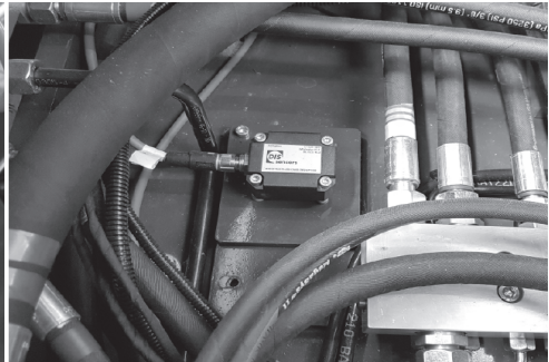
Fig. 23 Inwendige elektronische luchtbel
