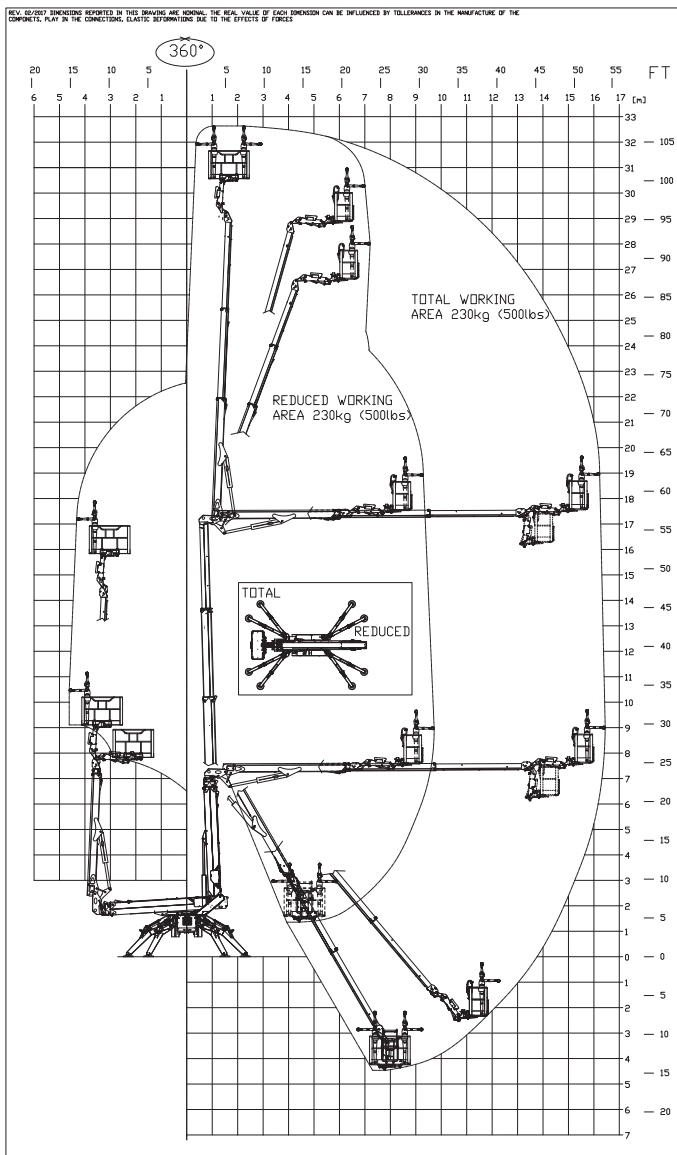
Fig. 63 Werkgebied
