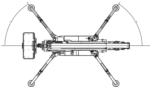
Fig. 74 STABILISATIEPOOT-Totaal gebied
