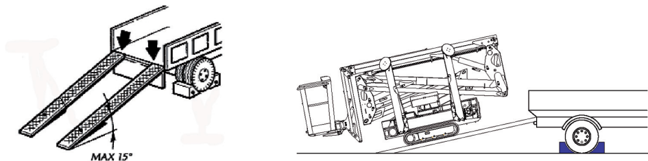
Fig. 139 Met oprijplanken laden
