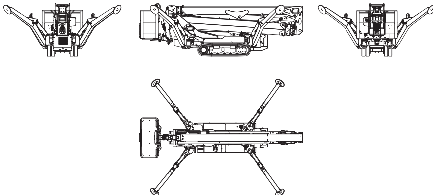
Fig. 71 Stabilisatiestand
