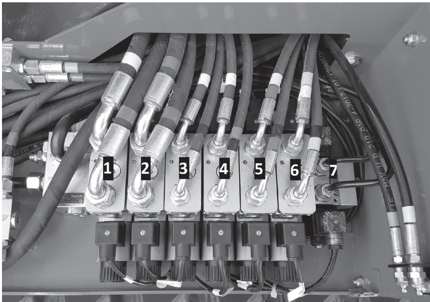
Fig. 133 Hydraulische verdeler grondgedeelte
