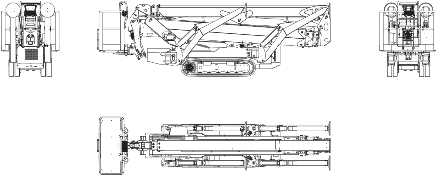
Fig. 70 Transportstand
